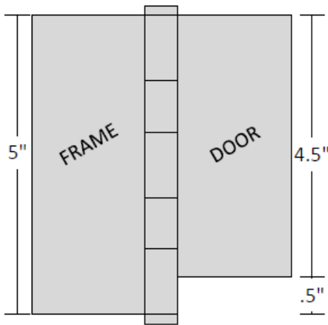
UNEQUAL BOTTOM (LH)
