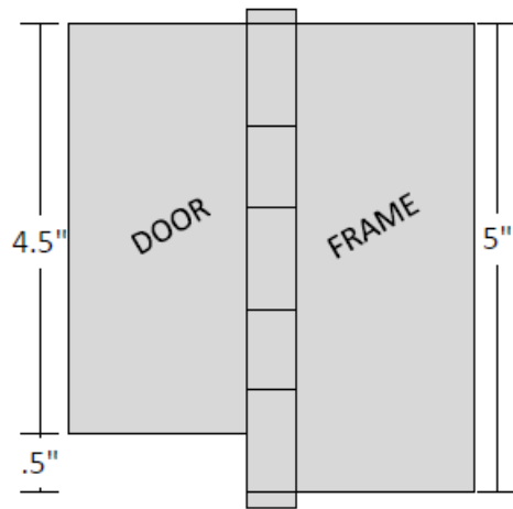
UNEQUAL BOTTOM (RH)
